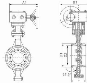
主要外形及连接尺寸(mm)
